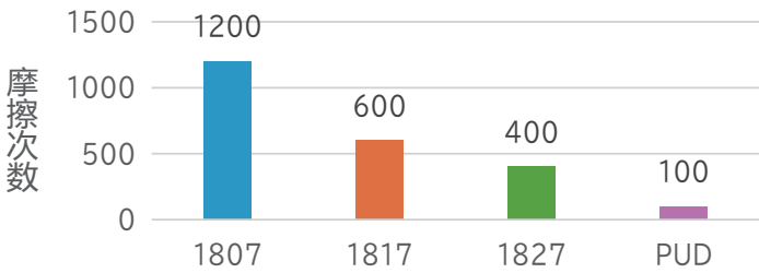
牢固度测试 (载荷4.9N、摩擦对象 棉布)
